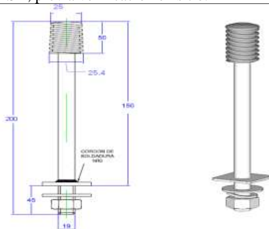
PERNO ESPIGA (PIN) TOPE DE POSTE SIMPLE ACERO GALVANIZADO 19 mm. DE DIÁM. X 450mm. DE LONG. CON ACCESORIOS DE SUJECCIÓN
