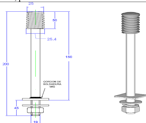
PERNO ESPIGA (PIN) TOPE DE POSTE SIMPLE ACERO GALVANIZADO 19 mm. DE DIÁM. X 450mm. DE LONG. CON ACCESORIOS DE SUJECIÓN
