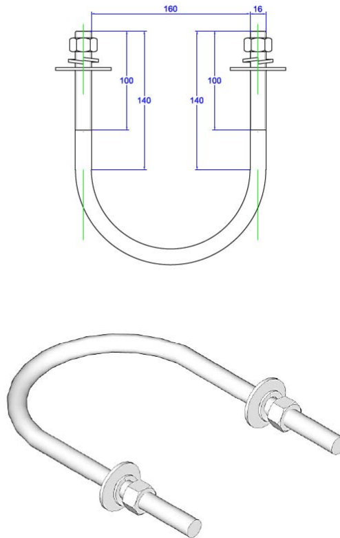
BRAZO DE ACERO GALVANIZADO TUBULAR PARA TENSOR FAROL 51 mm. X 1500 mm
